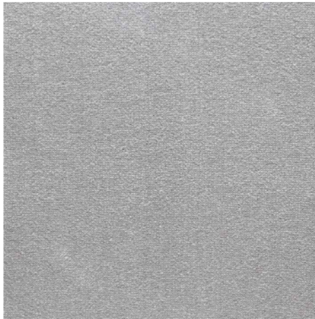
129 Venus
